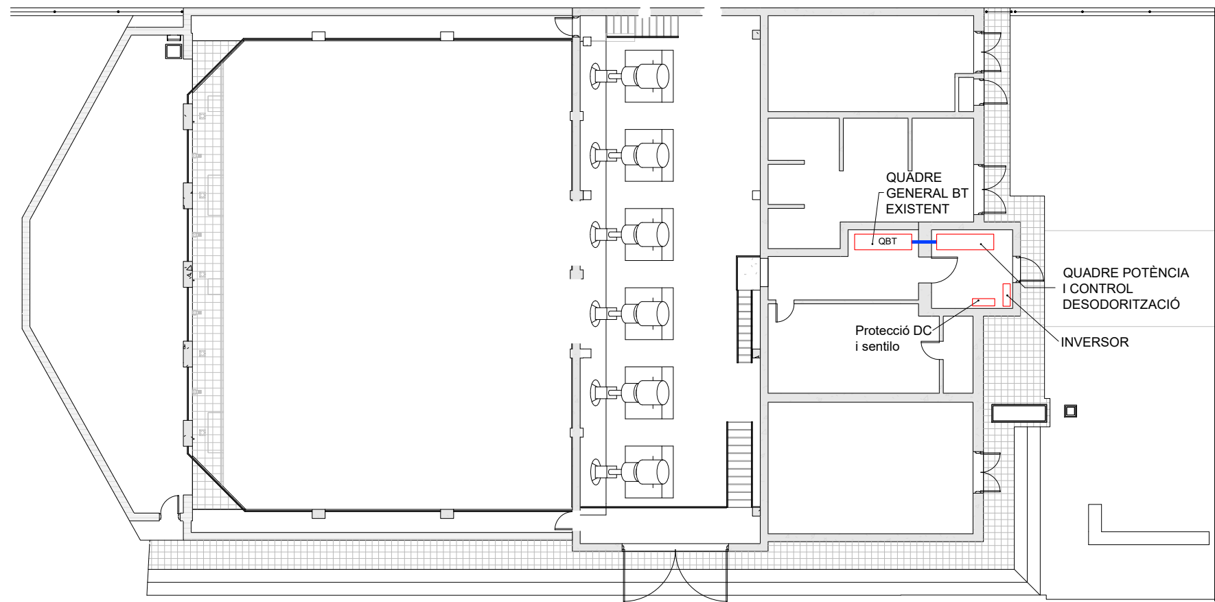
Planta nivell carrer E: 1/200
