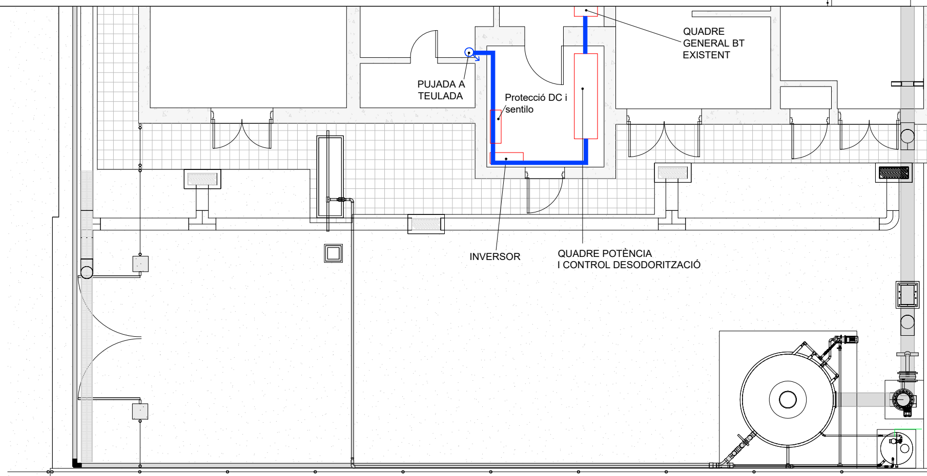
Planta nivell vorera E: 1/100
