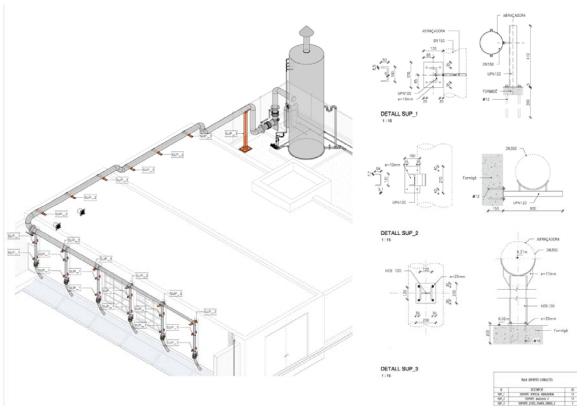
Imatge 13.- Traçat per coberta de la futura canonada de desodorització
