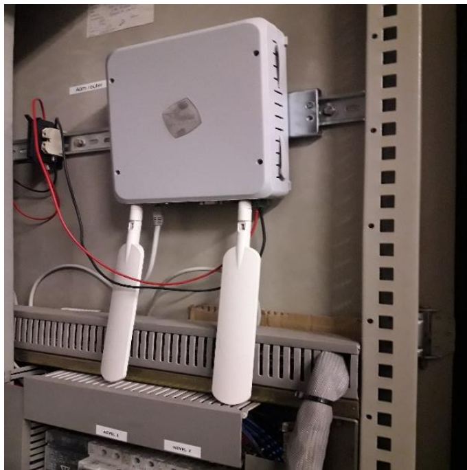
Imatge 15.- Router 3G de l'armari de comunicacions.
