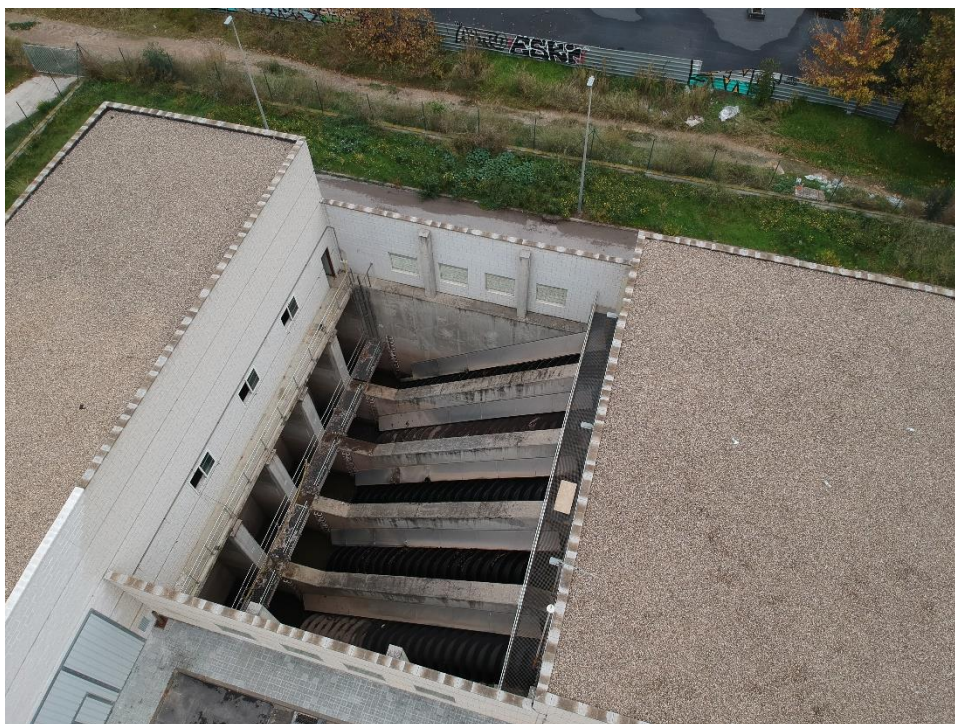
Imatge 7.- Vista coberta de l'edifici. Cargols d'Arquímedes
